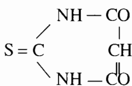
Thio uracil
